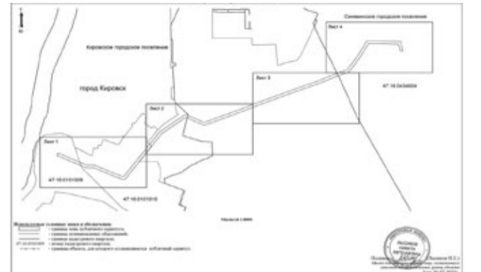
Схема расположения ВЛ 110 кВ Дубровская ТЭЦ - Северная птицефабрика (ВЛ 110 кВ Дубровская-9) Адрес: Ленинградская область, Кировский район, От ГРЭС-8 в г. Кировске на восток к ПС-390 около Птицефабрики Северная в 2 км южнее н.п. Синяино
